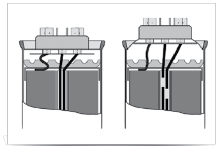
Abb.: Prinzip der Überdruckabreißsicherung
